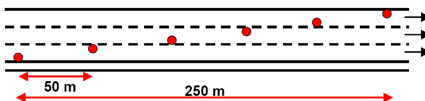
Esempio di schema di rilievo nel caso di intervento eseguito sull'intera carreggiata a 2 corsie
